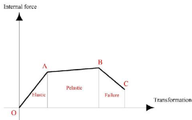
شکل ۱ - عضو شکل پذیر (شکست نرم)
